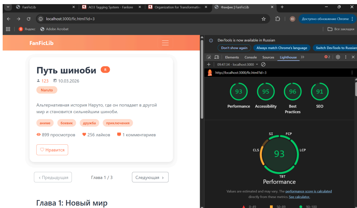
рис.1, Пример запуска тестов Lighthouse
